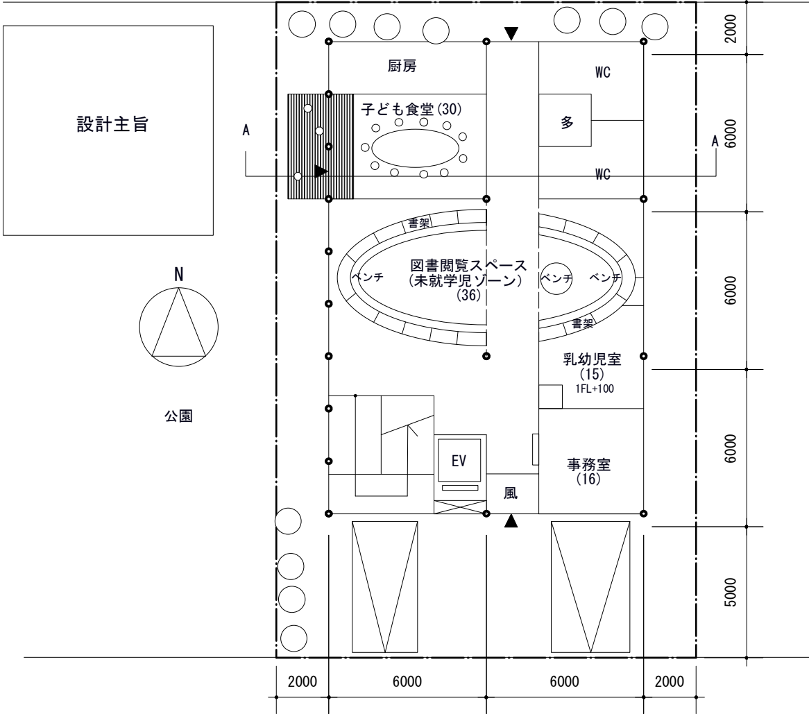
配置図兼1階平面図 S=1:100
