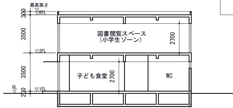
A-A断面図 S=1:100
