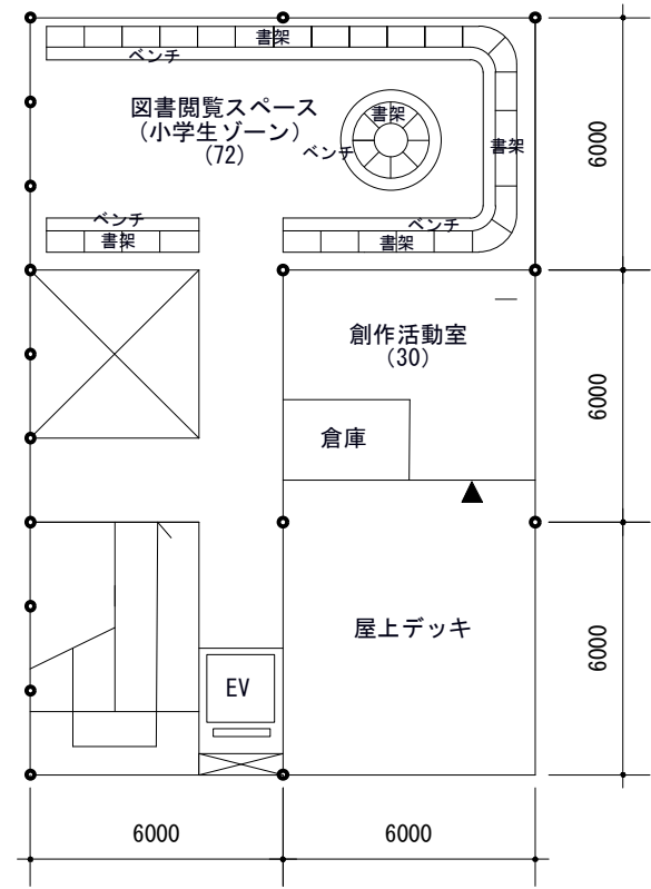
2階平面図 S=1:100
